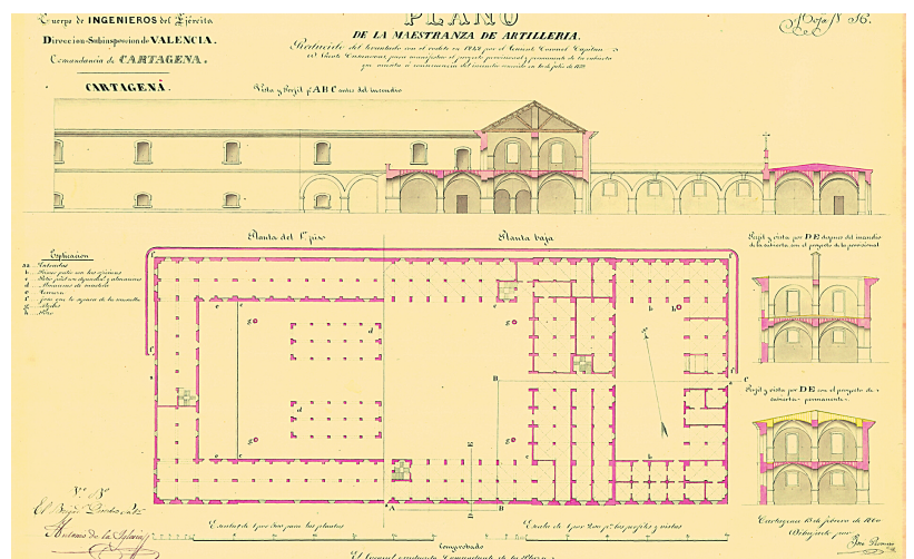
Plano de la Maestranza de Artillería realizado en 1860
